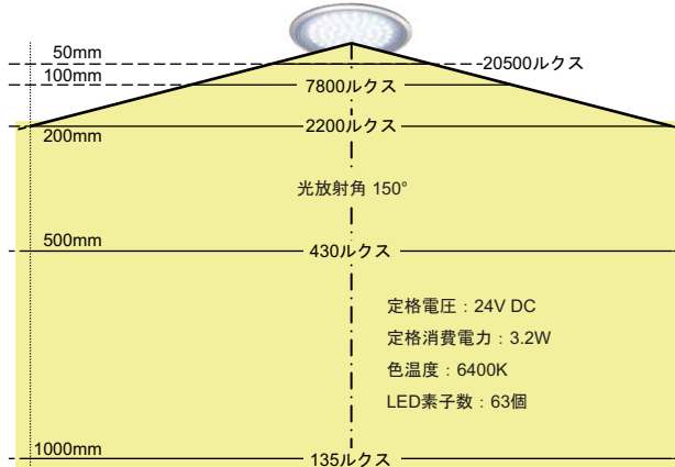
LD7003-78LV
