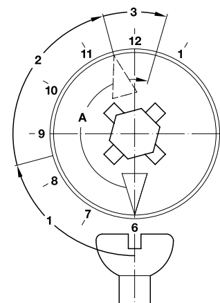
การทำงานของเกือกม้า MINIFIX ตามการหมุนของเข็มนาฬิกา
