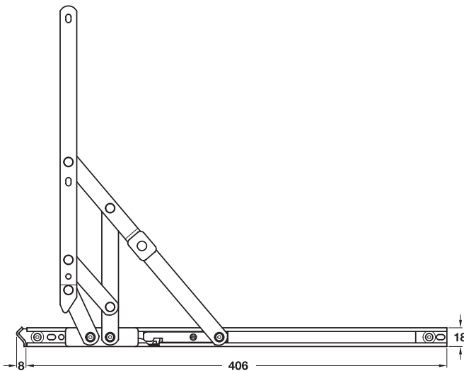
Side Hung บานพับหน้าต่างบานเปิด
