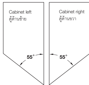
Base unit front extension, angled version (55°) ชุดตู้เตี้ยตั้งบานเปิด แบบเข้มนุม 55°
