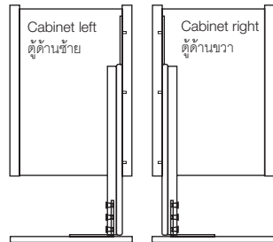
Base unit front extension, straight version (90°) ชุดตู้เตี้ยตั้งบานเปิด แบบตรง 90°
