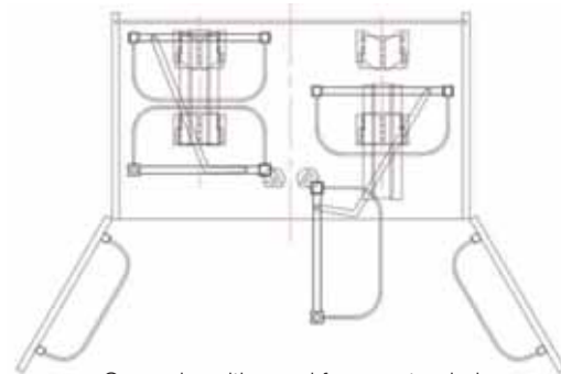
Opened position and frame extended ตำแหน่งตู้เปิดและเลื่อนเฟรม
