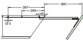
Base unit front extension, straight version (90°) ชุดตู้เตี้ยตั้งบานเปิด แบบตรง 90°
