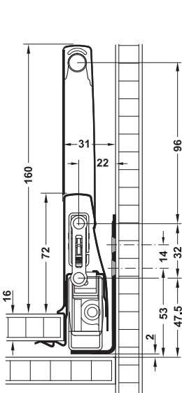
Drawer side height 92 mm แผงข้างสูง 92 มม.
