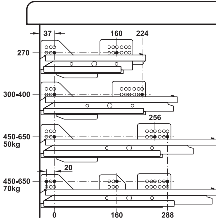
Drawer side height 92 mm ความสูงแผงข้างลิ้นชัก 92 มม.
