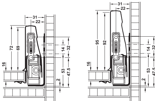
Drawer side height 92 mm ความสูงแผงข้างลิ้นชัก 92 มม.
