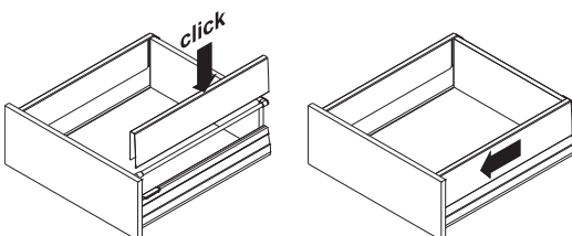
Drawer side height 92 mm แผงข้างสูง 92 มม.
