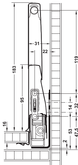
Drawer side height 115 mm แผงข้างสูง 115 มม.
