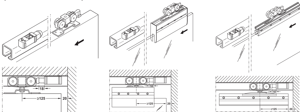
For sliding door fitting Classic 40-P/80P/120-P สำหรับรุ่น Classic 40-P/80-P/120-P
