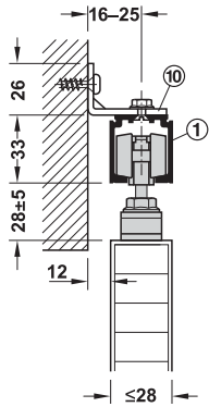
Wall mounting with wall mounting bracket การติดตั้งบนผนังด้วยเฟลทติดผนัง
