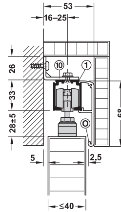
Wall mounting with mounting bracket and fixing clip for wooden panel การติดตั้งบนผนังด้วยเฟลทติดผนังและฝาปิดแบบคลิปสำหรับบานไม้
