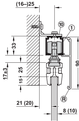
Wall mounting with wall mounting bracket and clip panel 90 mm การติดตั้งบนผนังด้วยเหล็กจากติดผนัง และฝาครอบรางแบบคลิก 90 มม.
