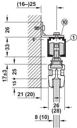
Wall mounting with wall mounting bracket การติดตั้งบนผนังด้วยเหล็กจากติดผนัง
