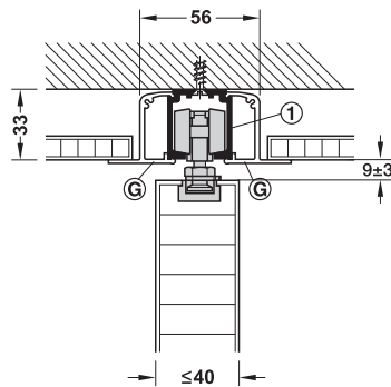
Ceiling installation with running track and 2xclip panel for integration in suspended ceilings การติดตั้งบนเพดานด้วยรางและฝาปิดพร้อมแผ่นปิดด้านล่าง
