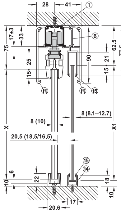
Ceiling installation with running track and clip panel 90 mm incl. fixed component. Sealing profile on one side for glass thickness 10 mm and wet sealing for glass thicknesses 8-12.7 mm การติดตั้งรางที่เพดานและฝาครอบราง 90 มม. พร้อมรางติดตายสำหรับกระจกบานหนา 10 มม. และสำหรับกระจกบานหนา 8-12.7 มม.
