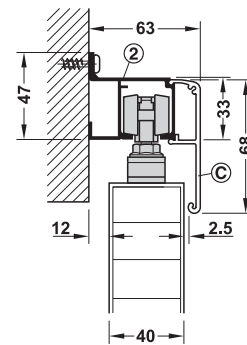
Wall mounting with running track and clip panel 68 mm การติดตั้งบนผนังด้วยอุปกรณ์หุ้มรางติดผนังและฝาปิดแบบคลิป 68 มม.
