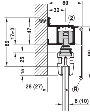
Wall mounting with running track and clip panel 90 mm การติดตั้งบนผนังและฝาครอบราง แบบคลิก 90 มม.
