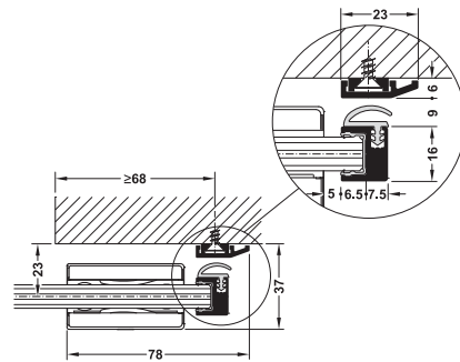
End profile wall installation include rubber seal ติดตั้งบานเลื่อน
