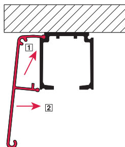
First click into position 1, than to position 2 ติดตั้งเข้าในตำแหน่งที่ 1 ก่อน จากนั้นกดเข้าไปยึดในตำแหน่งที่ 2
