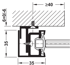
Wall profile set include rubber seal การติดตั้งรางซีลที่ผนัง
